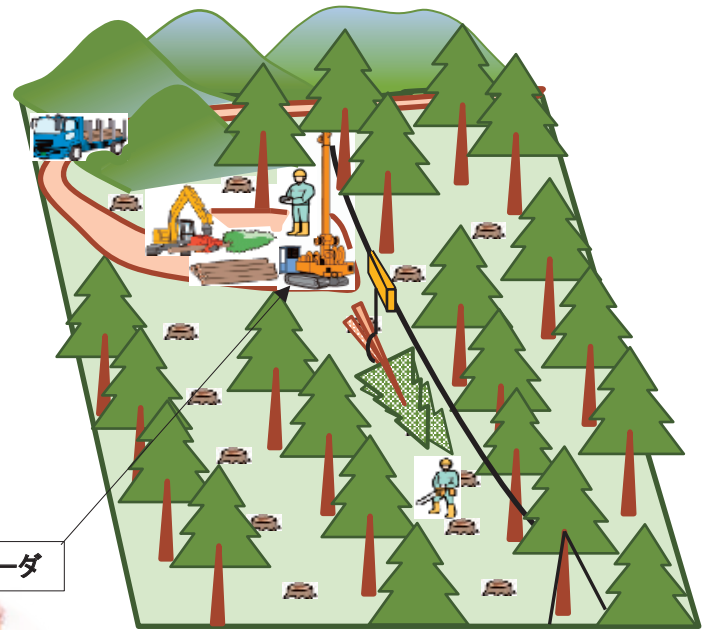
タワーヤーダを活用した架線系集材のイメージ図。（列状間伐） 例：斜面下方の伐倒木を斜面上方のタワーヤーダで引っ張り上げる。
